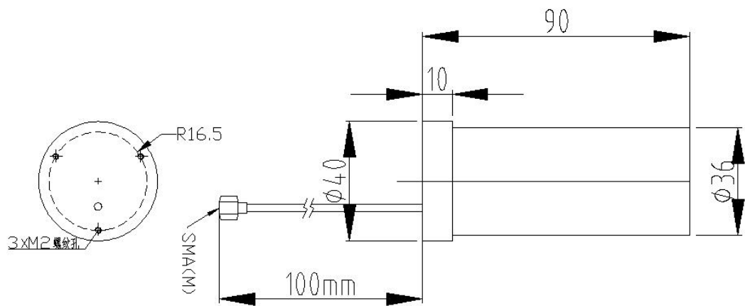
图1 天线结构尺寸图
