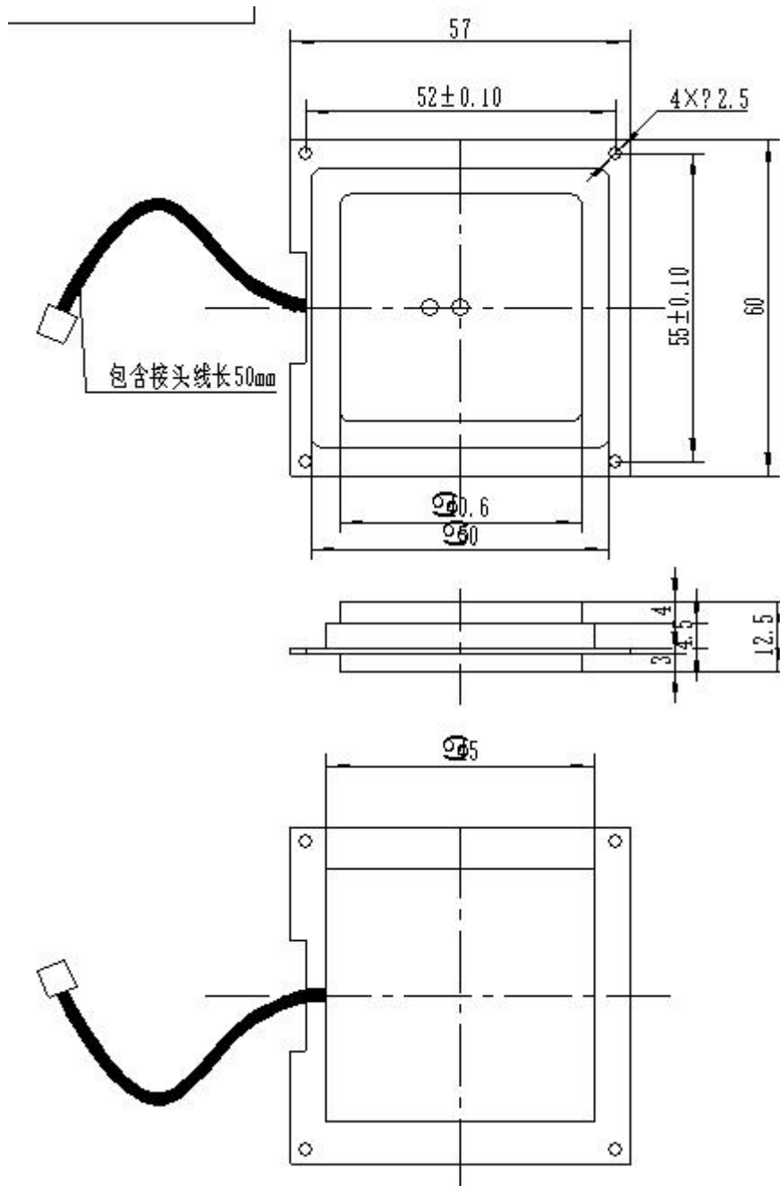
图1 天线结构尺寸
