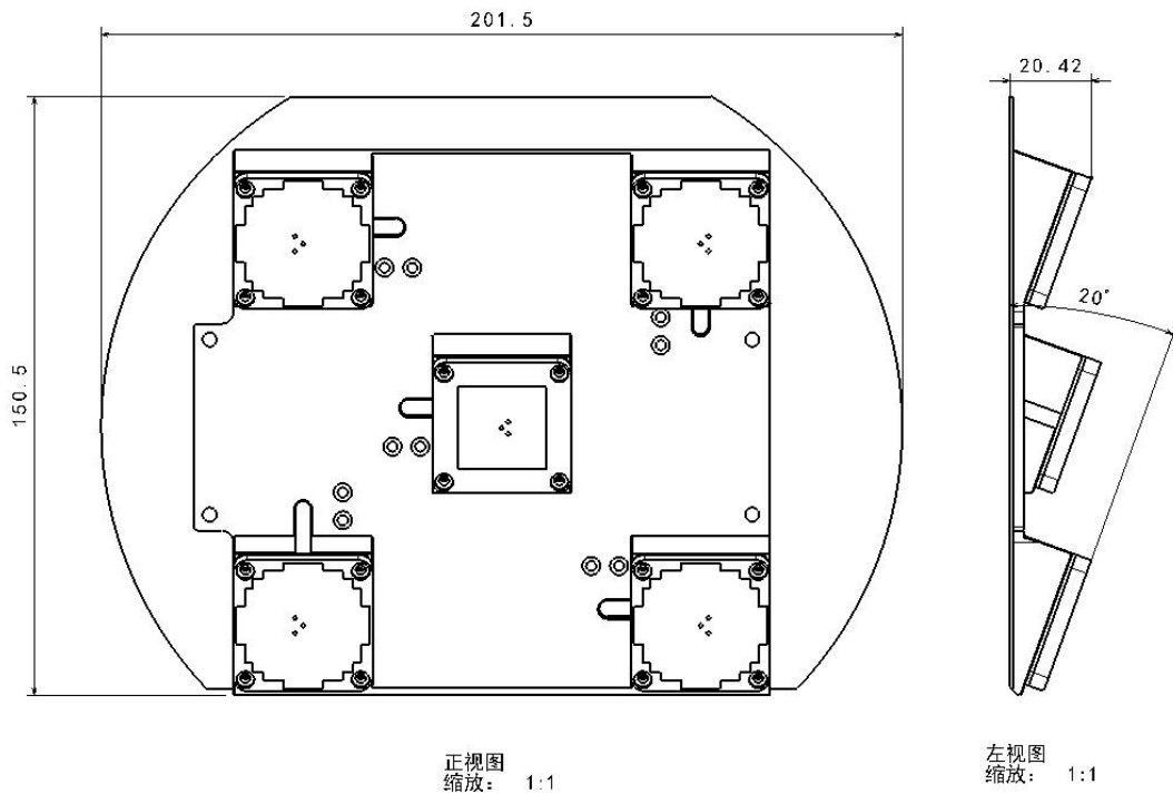
图1 天线结构尺寸图
