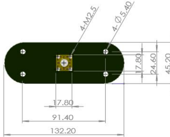
设备外廓尺寸和安装形式
