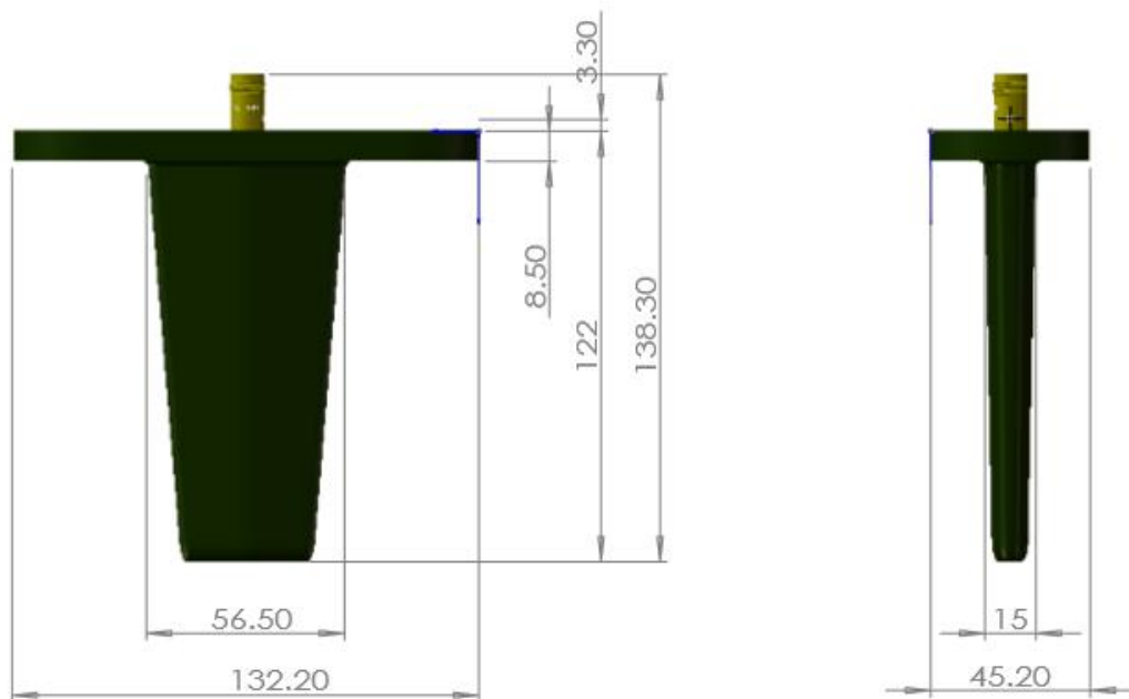
机载天线外廓尺寸
