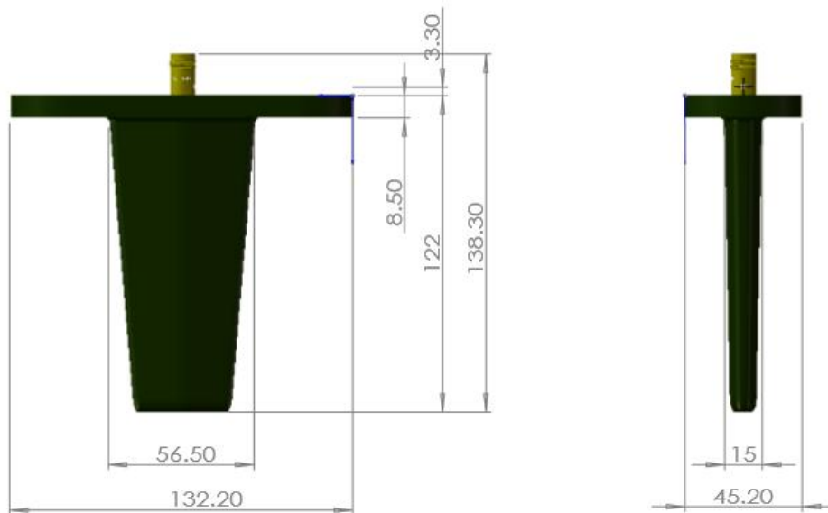
机载天线外廓尺寸
