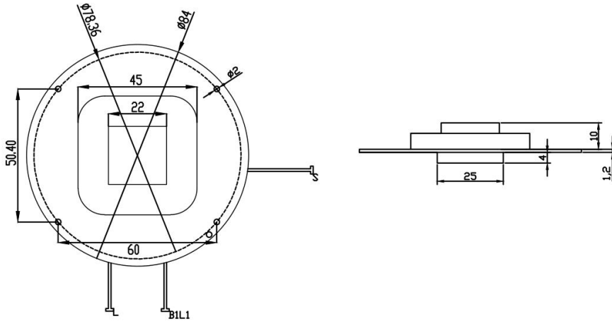
图1 天线尺寸图
